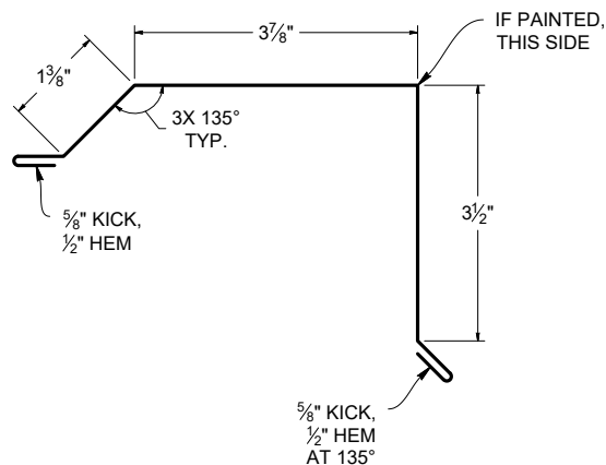
MODIFIED MINI GABLE ( T3MMG )
